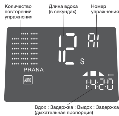
Рис. 4c Дисплей дихального тренажера PRANA (на примере PRANA AUTO)
